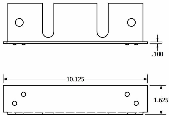
Jamb Clips (12ga Galvaneal)
